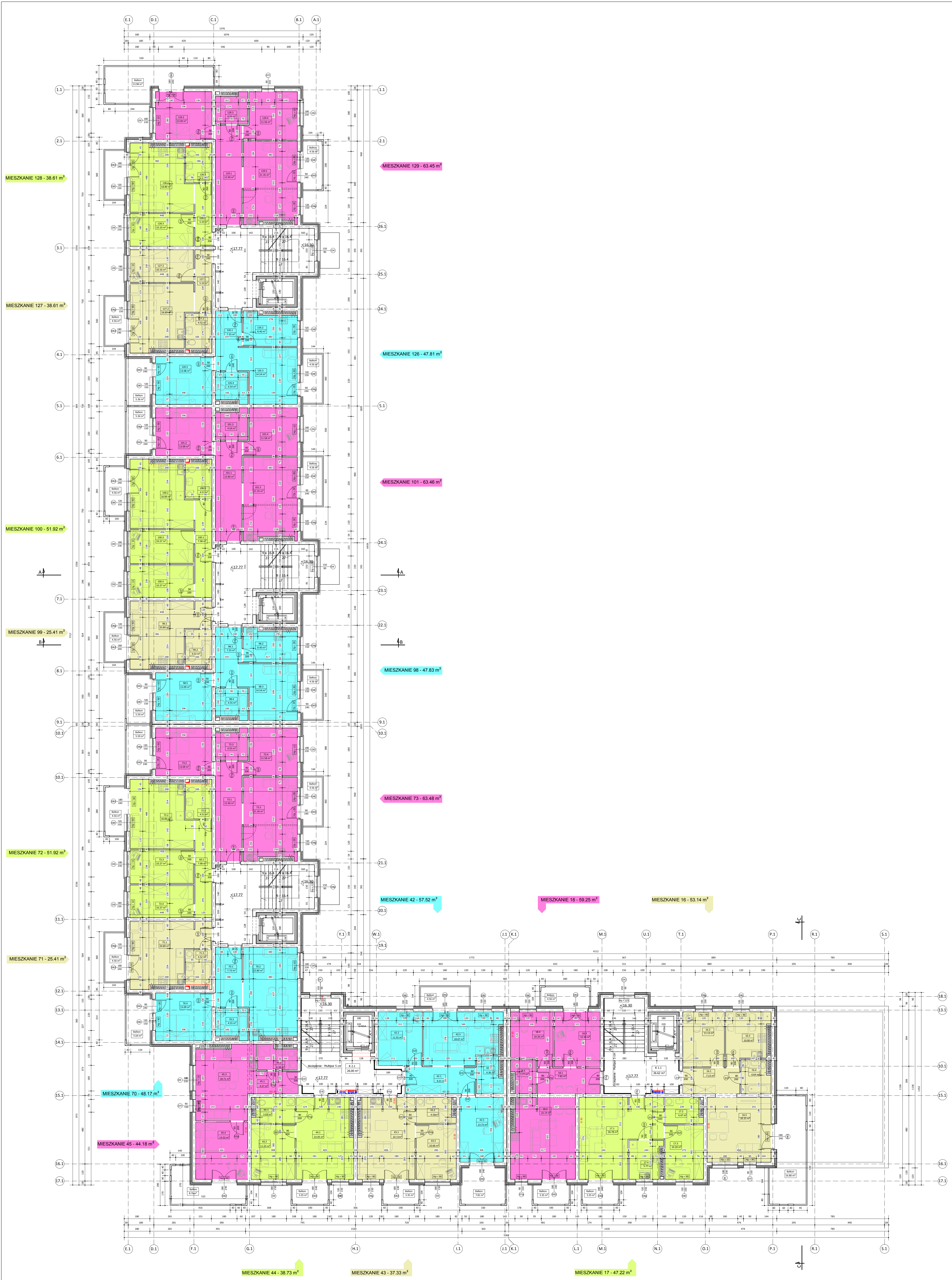
BUDYNEK B - RZUT VI PIĘTRA
