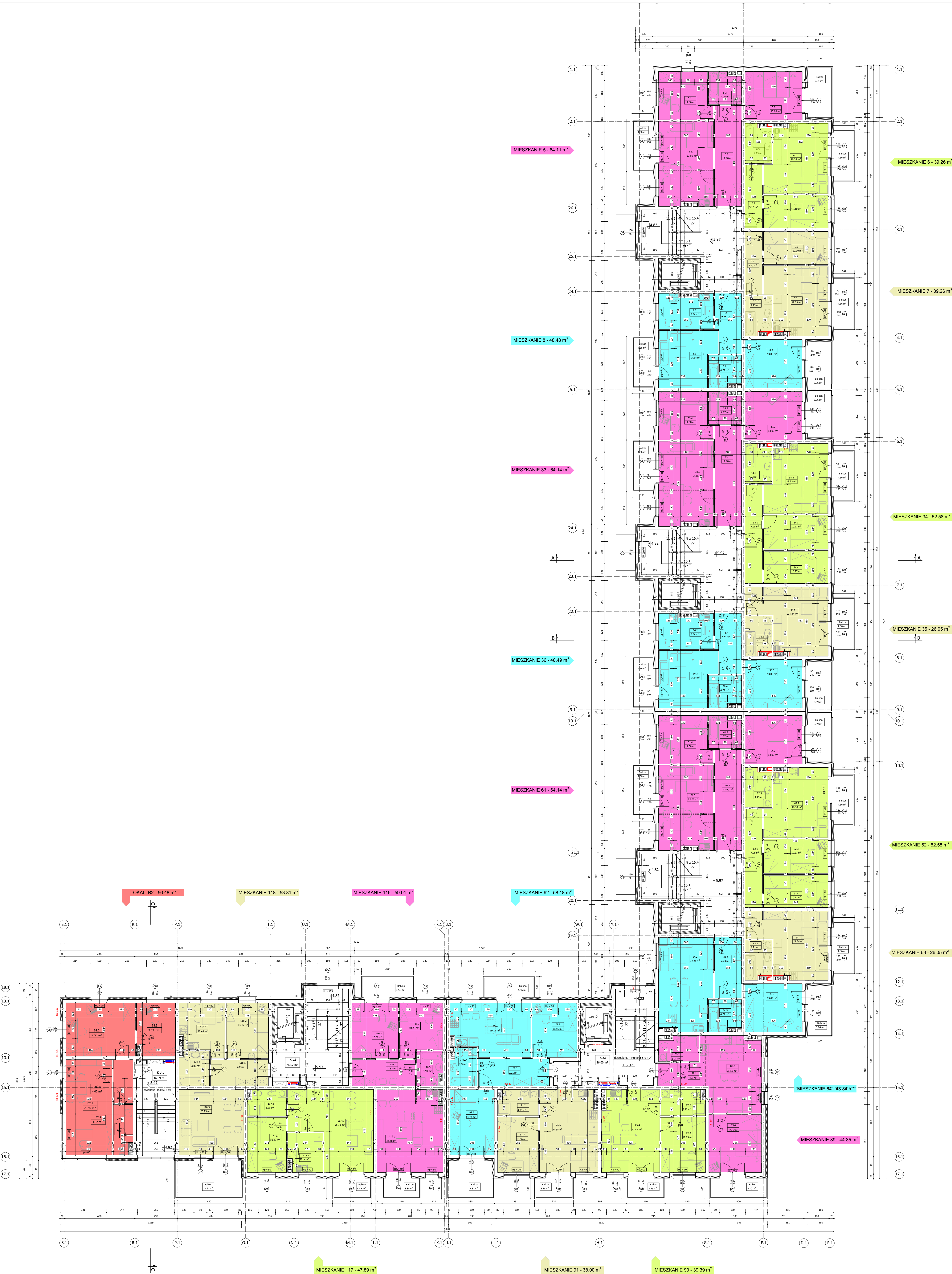
BUDYNEK A - RZUT II PIĘTRA
