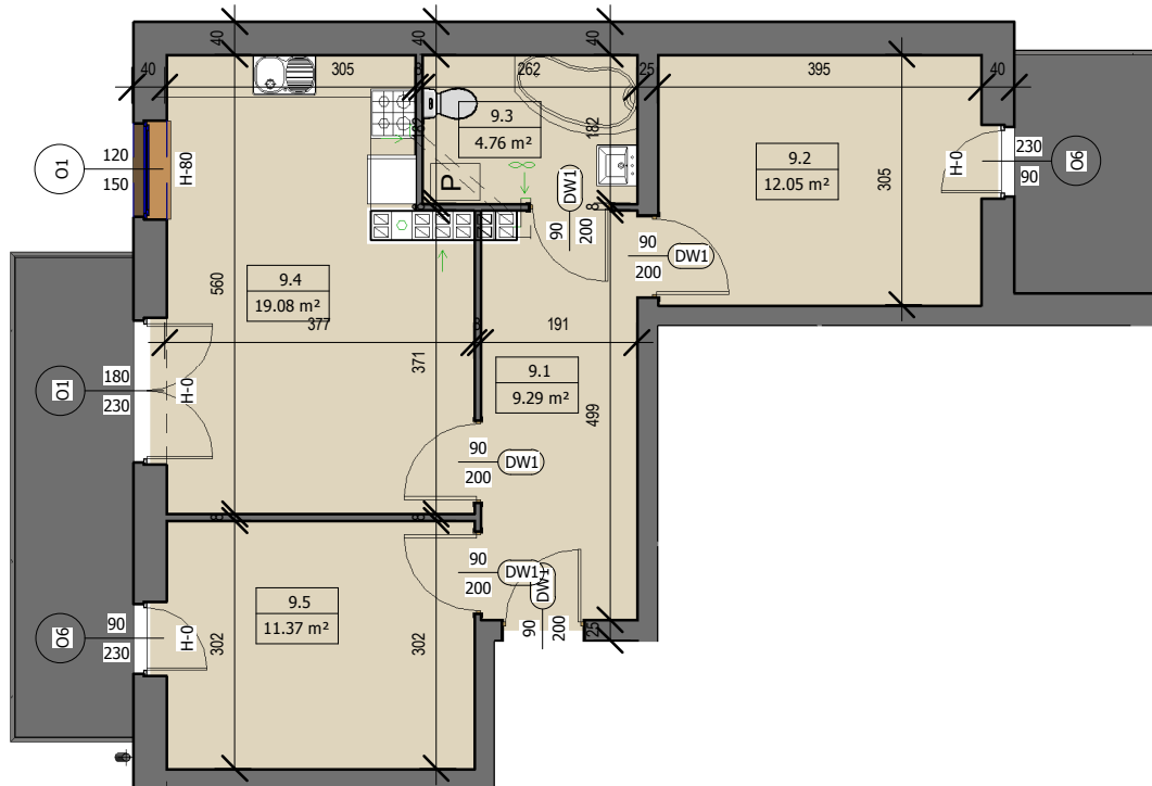
Rzut mieszkania skala 1:100
