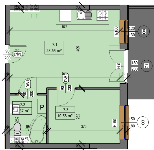
Rzut mieszkania skala 1:100
