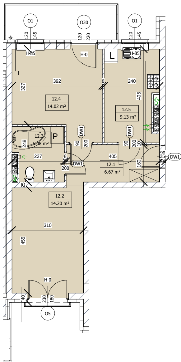
Rzut mieszkania skala 1:100
