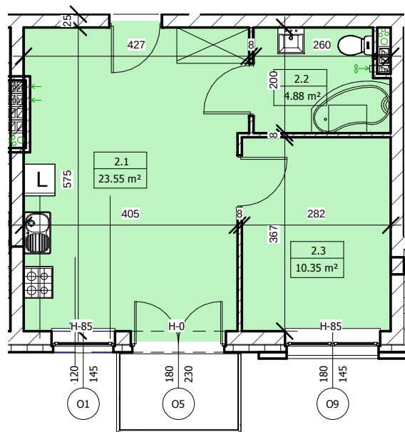
Rzut mieszkania skala 1:100
