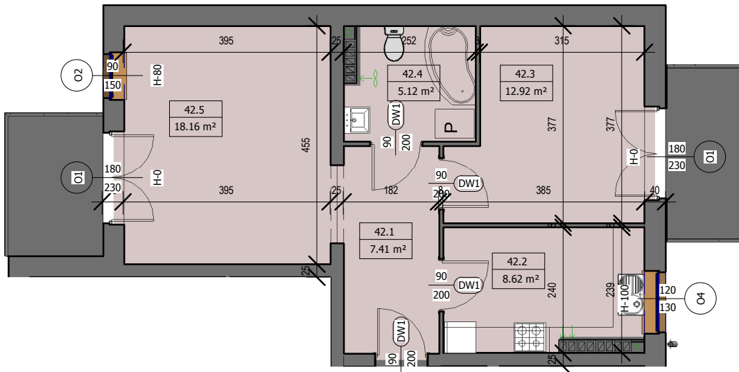
Rzut mieszkania skala 1:100
