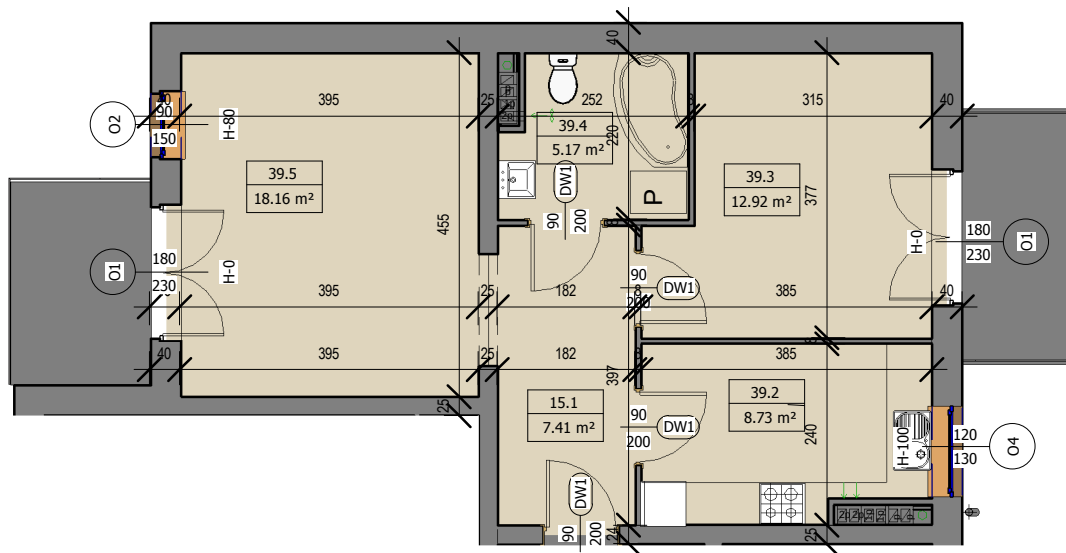
Rzut mieszkania skala 1:100
