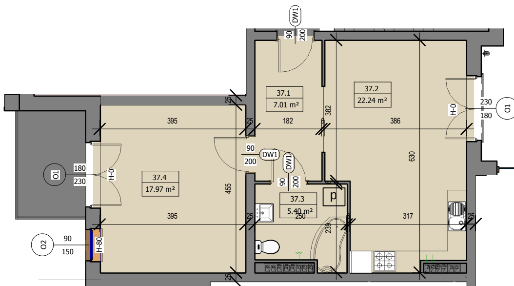
Rzut mieszkania skala 1:100
