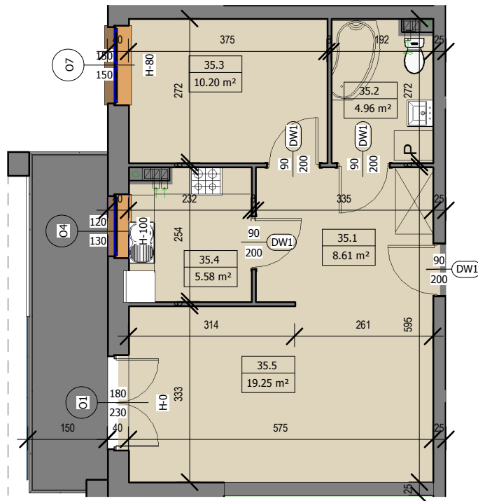
Rzut mieszkania skala 1:100
