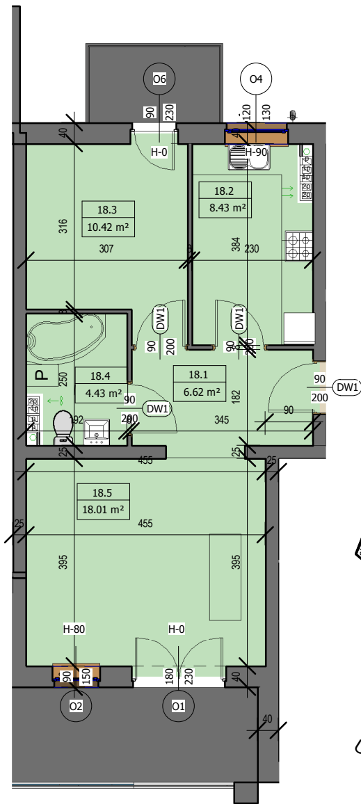
Rzut mieszkania skala 1:100
