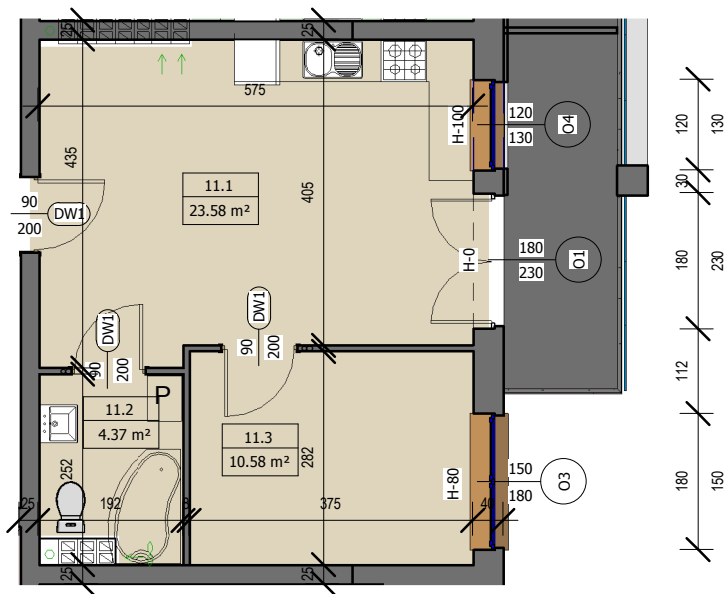
Rzut mieszkania skala 1:100
