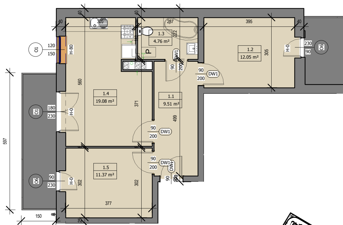
Rzut mieszkania skala 1:100
